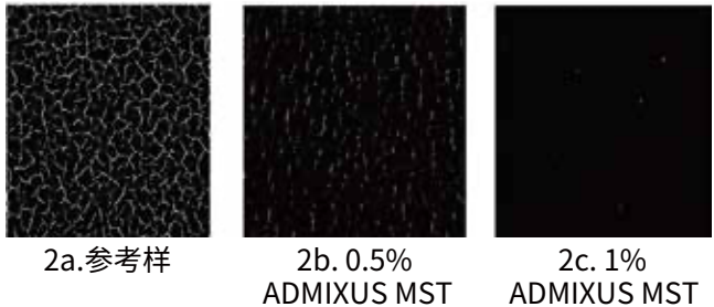
图 2 ❖ 数码照片显示，由于成膜不良，出现了不同数量的裂缝。
