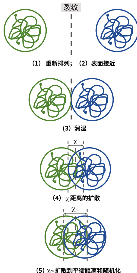
图1 ❖ 聚合材料中裂纹愈合的阶段。 5
