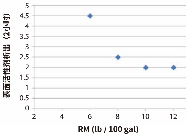
图 15 ❖ HEUR增稠剂用量对表面活性剂析出的影响。
