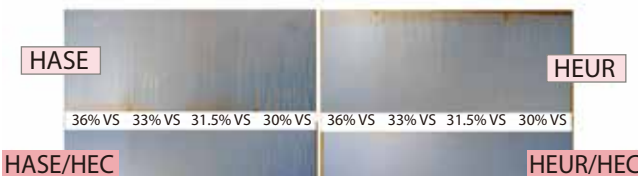
图 16 ❖ 在含HEUR/HASE增稠剂的涂料中添加HEC以改善表面活性剂的析出。
