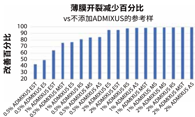
图3 ❖ 以改进为序，在55°F温度下固化，裂纹区域的减少(%)。在115°F下固化的沥青薄膜的拉伸性能。
