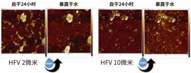
图 8 ❖ 暴露于水滴之前和之后，在室温下干燥的涂料表面的2D原子力显微镜相位图。亮色区域对应水溶性或无机材料（例如颜料）。较暗的区域对应于乳液聚合物。左图：突出显示了水溶性物质溶解的图像。右图：突出显示了从涂层主体到空气界面的物质提取。
