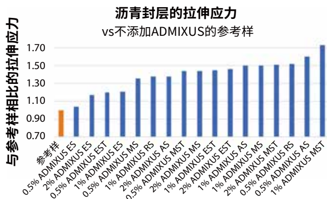
图6 ❖ 以极限应力增加为序，沥青薄膜（不含纤维参考样）的相对极限拉伸应力。
