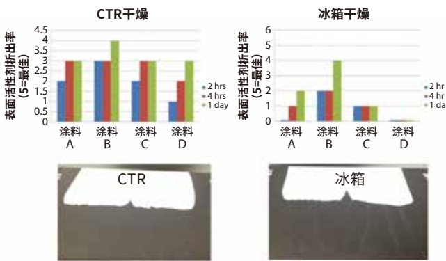
图 12 ❖ 干燥条件对表面活性剂析出的影响。左图：在CTR中进行干燥的样板。右图：在冰箱里进行干燥的样板。
