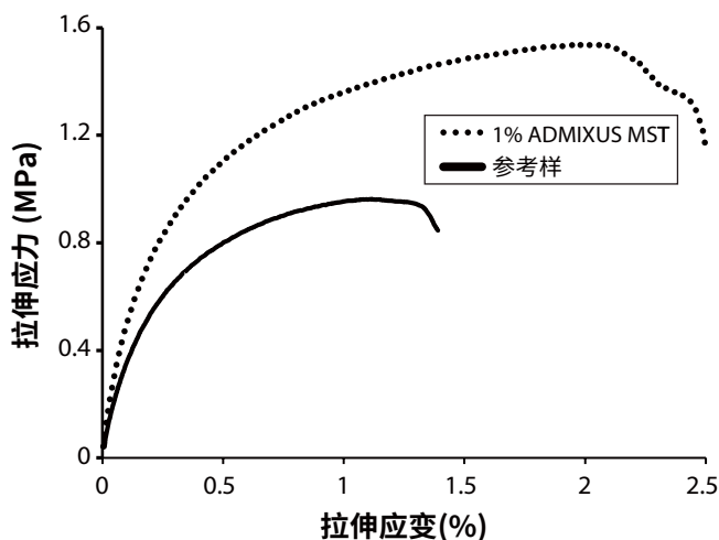
图4 ❖ 沥青薄膜试样的典型拉伸应力/应变关系 (a) 无纤维参考样和 (b) 添加了1% ADMIXUS MST，在115°F温度下固化。
