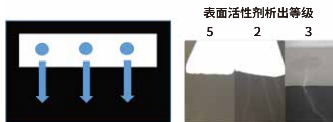
图3 ❖ ASTM 7190表面活性剂析出水条纹测试。
