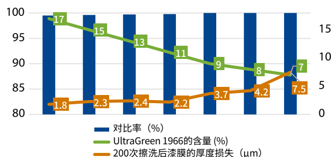
图1 ◆ 与新乳液含量相关的耐湿擦洗性。
