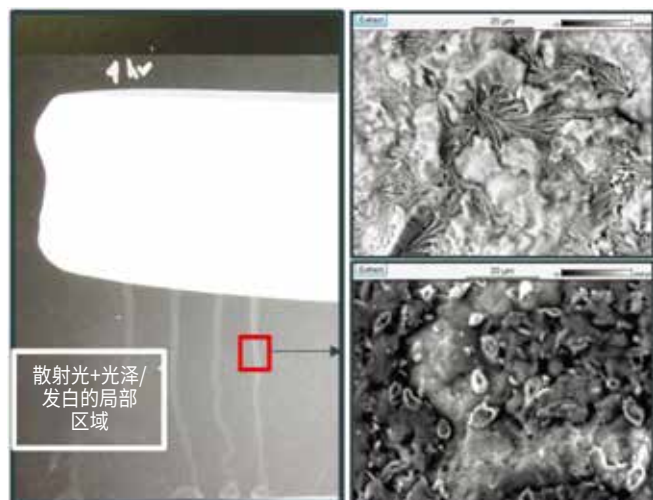
图4 ❖ 左图：光学图像显示了表面活性剂从白色涂层中渗出到黑色基材上。右图：扫描电子显微照片显示了两种不同类型的晶体形成。
