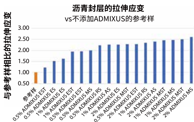
图5 ❖ 以极限应变增加为序，沥青薄膜（不含纤维参考样）的相对极限拉伸应变。
