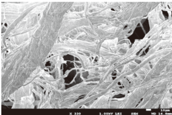
图1 ❖ 原纤化HDPE纤维的显微照片（由三井化学公司提供）。 3
