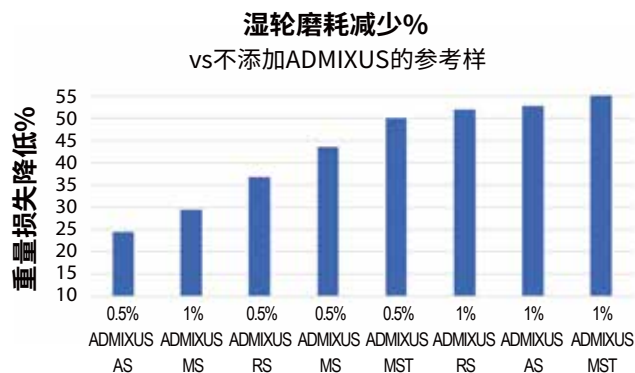
图8 乳化沥青薄膜的湿轮磨耗结果。 4
